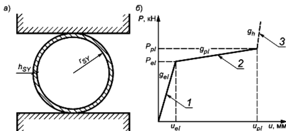
а - общий вид; б - диаграмма деформирования податливой опоры; 1 - упругая стадия; 2 - пластическая стадия; 3 - стадия отвердения; g_{el} - жесткость податливой опоры в упругой стадии деформирования; u_{el} - предельная деформация податливой опоры в упругой стадии; g_{pl} - жесткость податливой опоры в пластической стадии; u_{pl} - предельная деформация податливой опоры в пластической стадии
