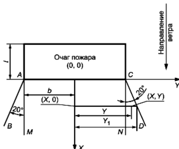
Рисунок Е.1 - Схема определения размеров зон загазованности от отдельного очага при направлении ветра перпендикулярно к фасаду здания
