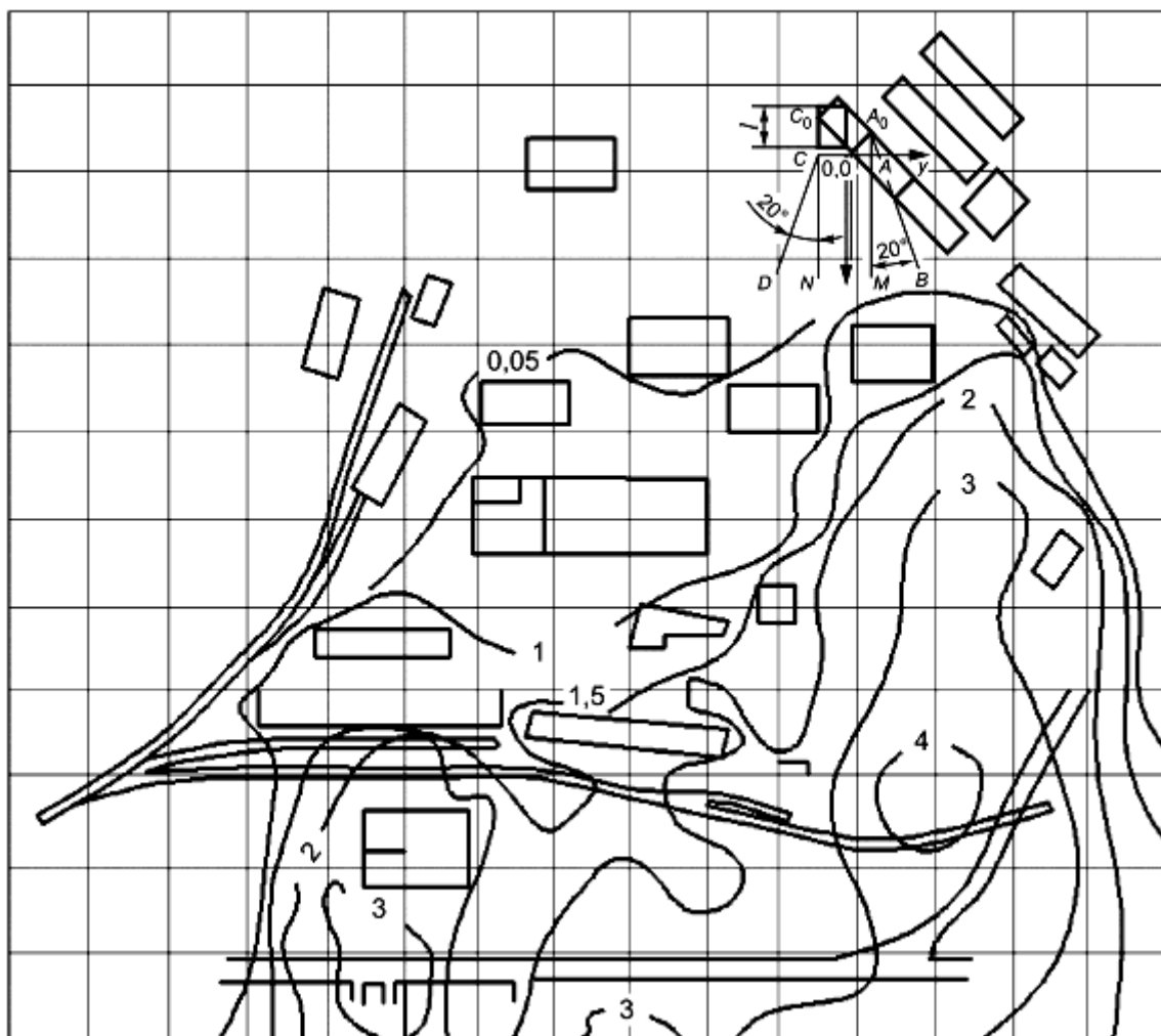
Рисунок Е.3 - Схема определения размеров зон загазованности для разных очагов пожара Е.1.6 При заданном месте расположения убежища концентрацию загазованности определяют только в одной точке - в месте расположения воздухозаборного устройства. При этом загазованность учитывают только от тех очагов пожара, в секторе которых находится убежище (в секторе, ограниченном лучами АВ и CD, см. рисунки Е.2 и Е.3). Приложение Ж
