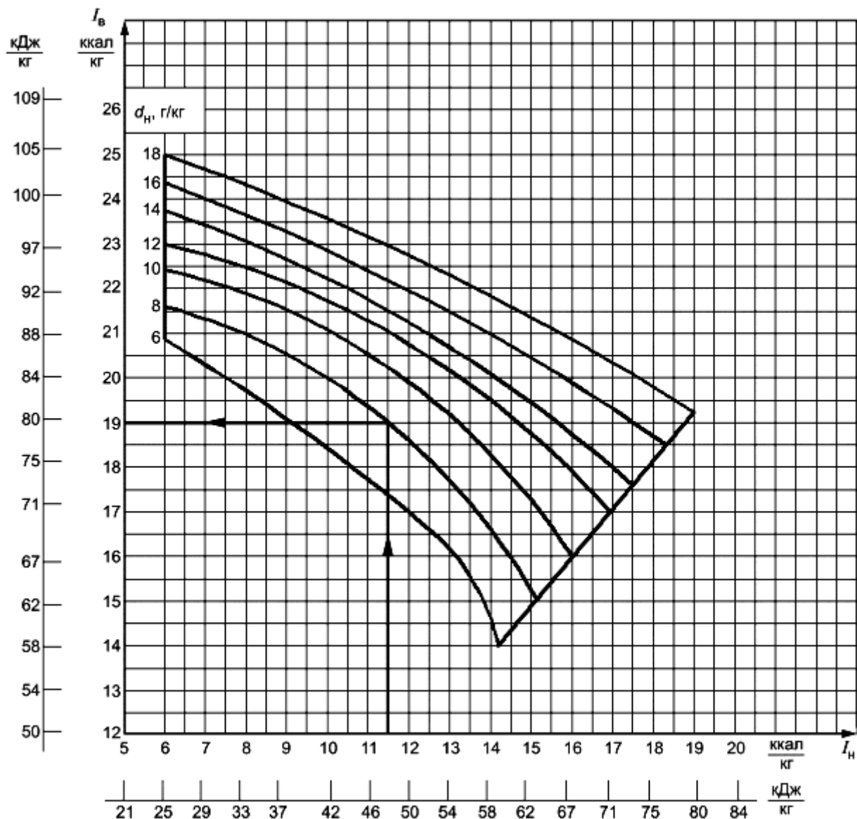
Рисунок Д.2 - Определение теплосодержания (энтальпии) внутреннего воздуха при удалении тепловых избытков системой вентиляции в режиме I и допустимых сочетаний температуры и влажности этого воздуха в третьей и четвертой климатических зонах
