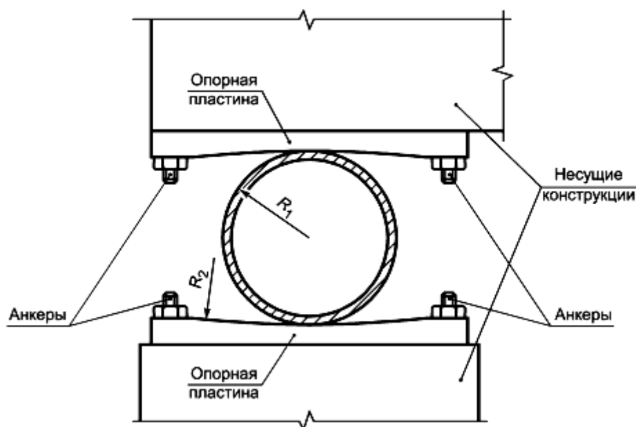
Рисунок 5.4 - Принципиальная схема устройства узла с податливой опорой
