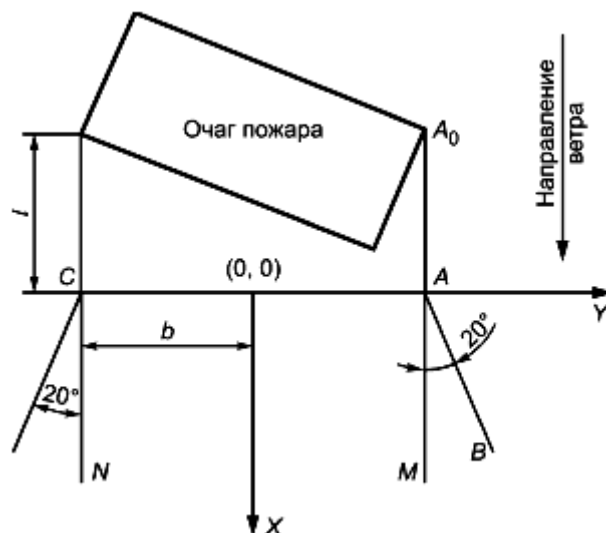
Рисунок Е.2 - Схема определения размеров зон загазованности от отдельного очага пожара при направлении ветра под острым углом к фасаду здания
