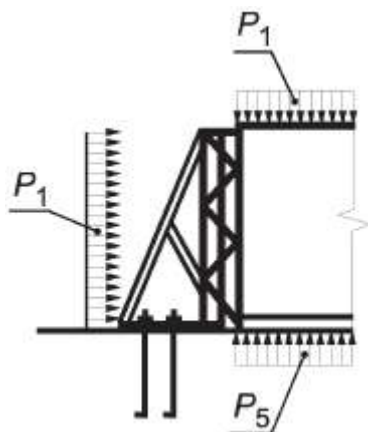
Рисунок 9.2 - Схема приложения динамической нагрузки на конструкции быстровозводимых убежищ
