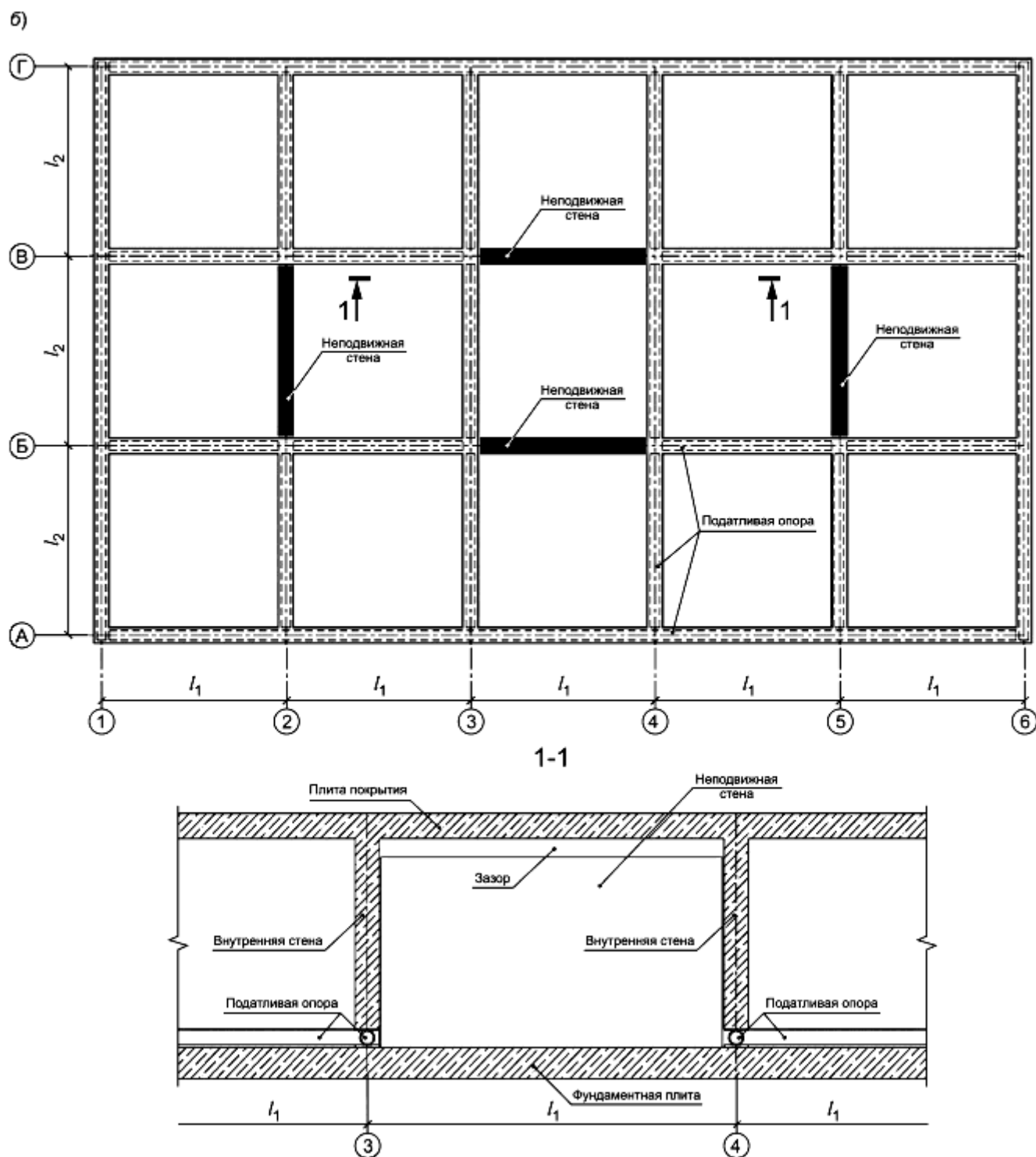
Рисунок 5.3 - Схема расстановки податливых опор и неподвижных стен для восприятия горизонтальной динамической нагрузки
